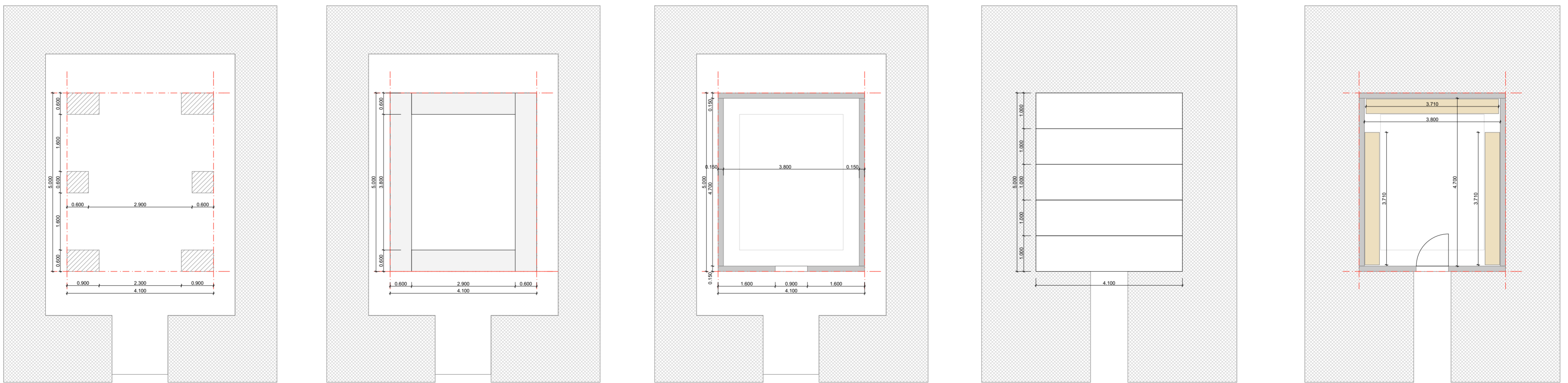
Plan toit
